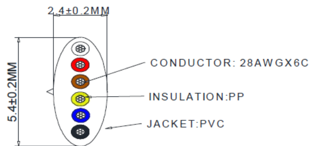
6P6C仕様のケーブル例
